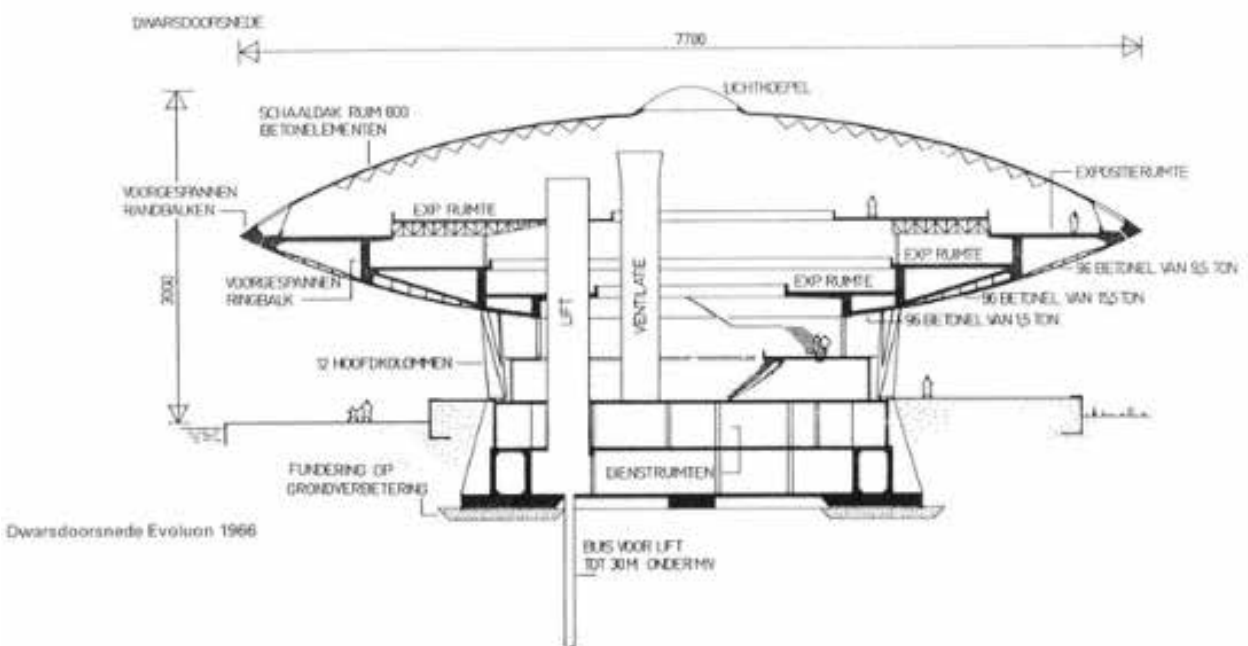
▲ Dwarsdoorsnede Evoluon. © Uit: Ir. Louis C. Kalf/Het artistieke geweten van Philips/Peter van Dam
